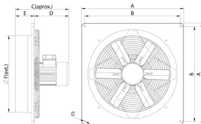
Διαστάσεις ΗJBM (mm)
