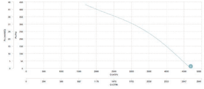
1 HJBM 35 T2 0,55kW
